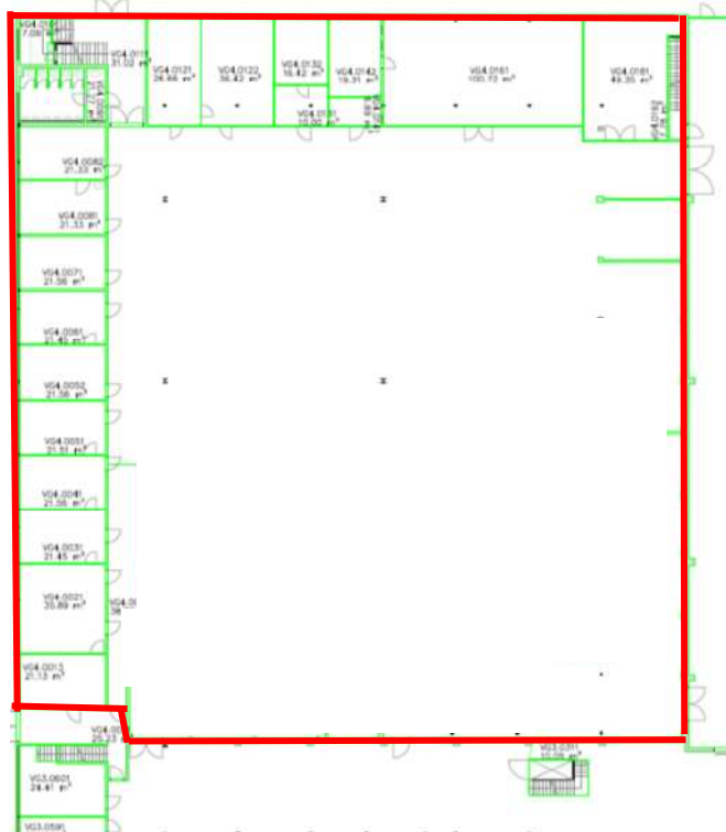
Erdgeschoss
